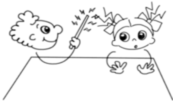
Статическое электричество
