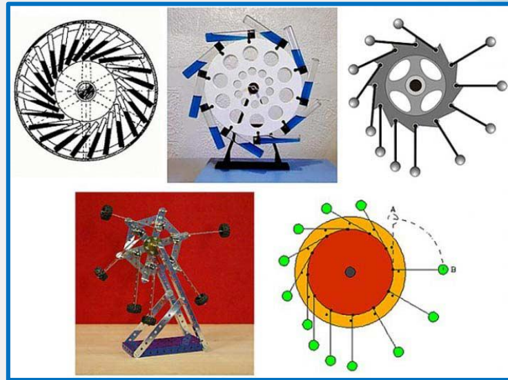
Вечный двигатель
