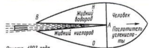
Ракета. 1903 года
