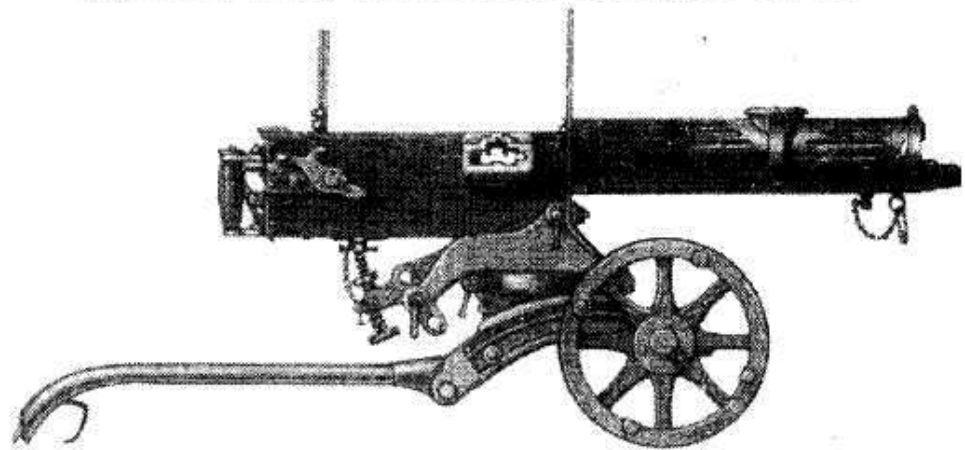
7,62 станковый пулемет Максима образца 1910 г.
