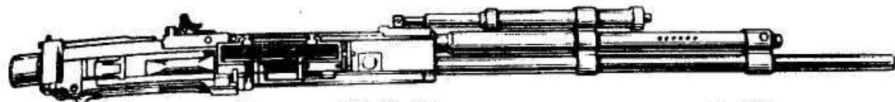
Авиационный пулемет УБ-12,7 (выпускался также заводом № 385).
